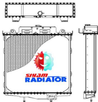
PT-018-SS
